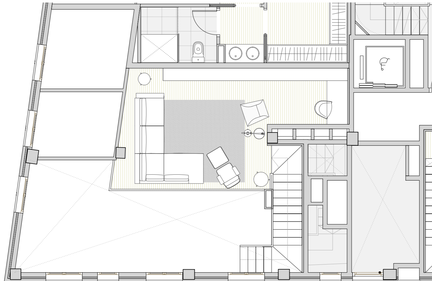
Planta Altell
